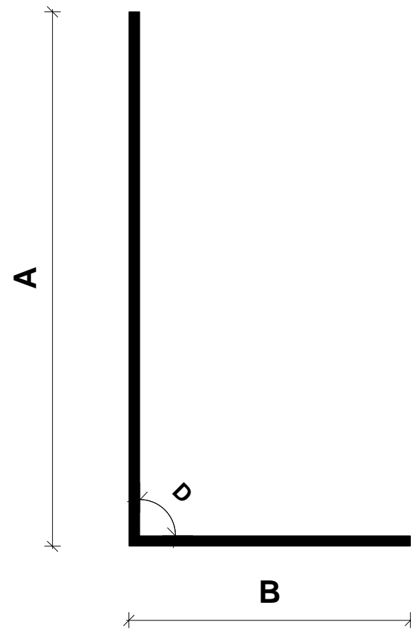
L-Profil 1 1:1
