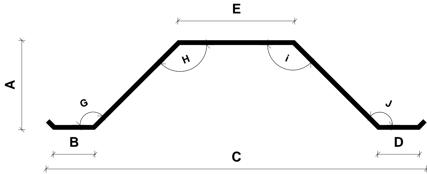
Hat Profil 3 1:1
