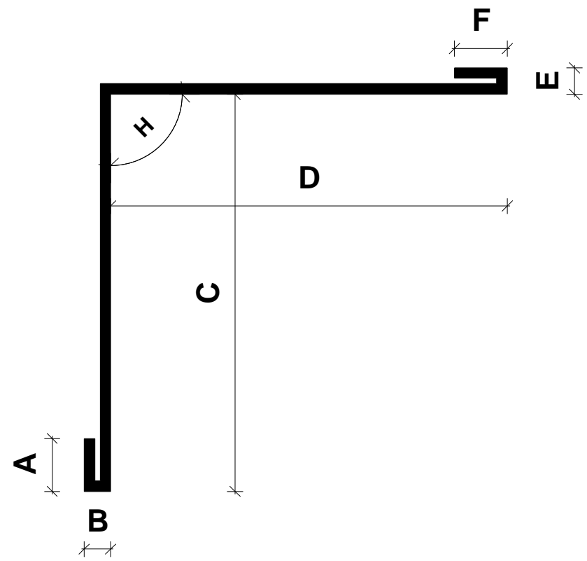
Hjørne Profil 4 1:1
