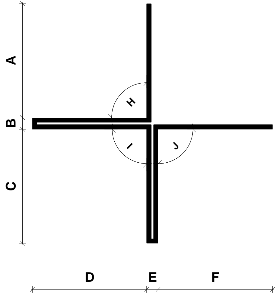
Hjørne Profil 3 1:1
