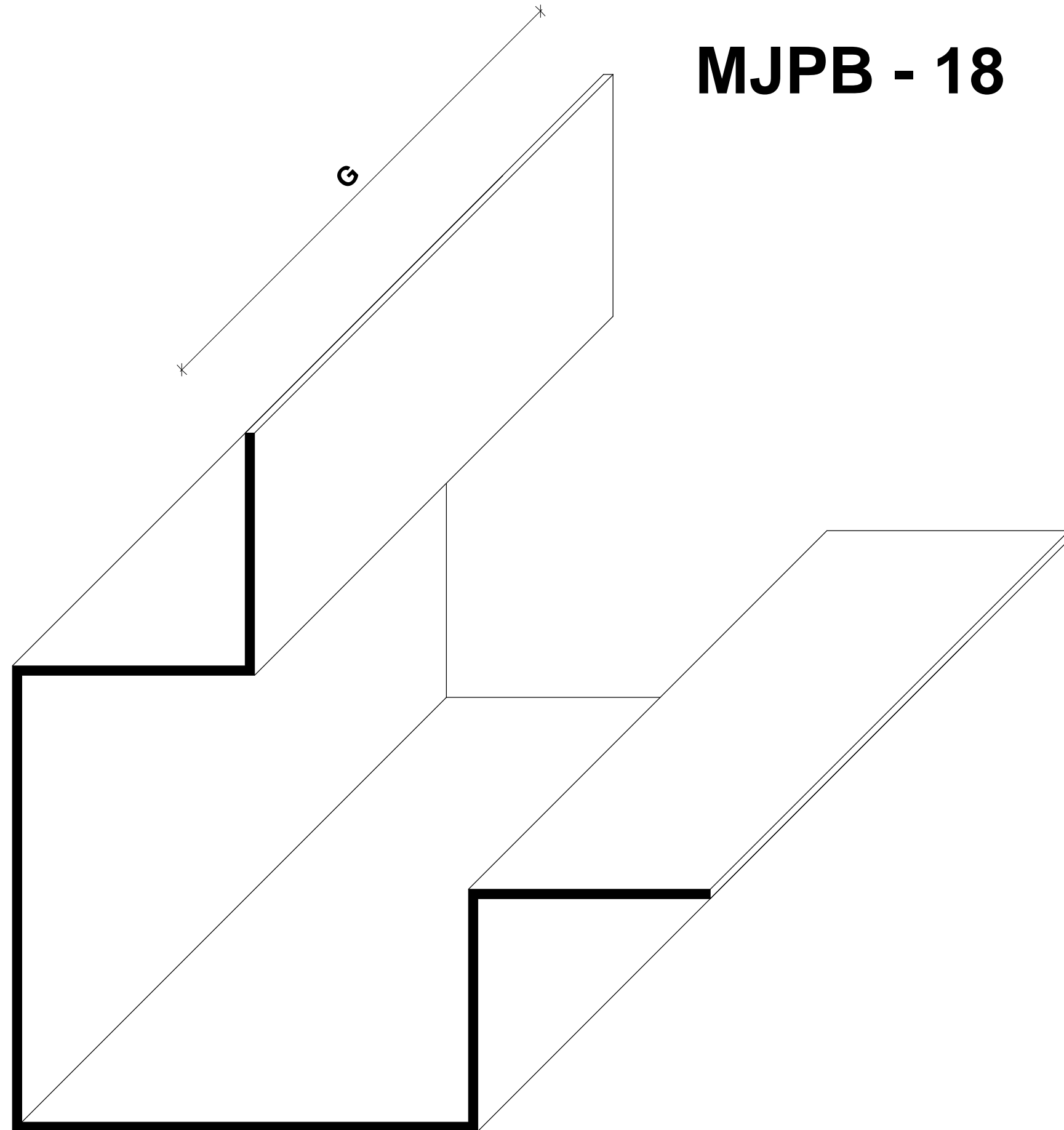
Hjørne Profil 1 3D
