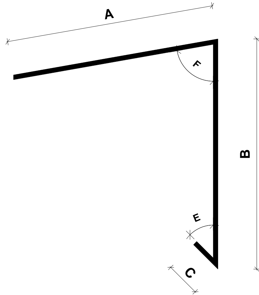
Vindskede 1 1:1
