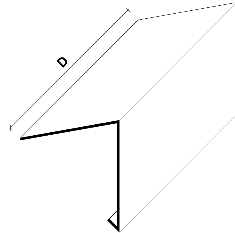
Vindskede 1 3D 1:2
