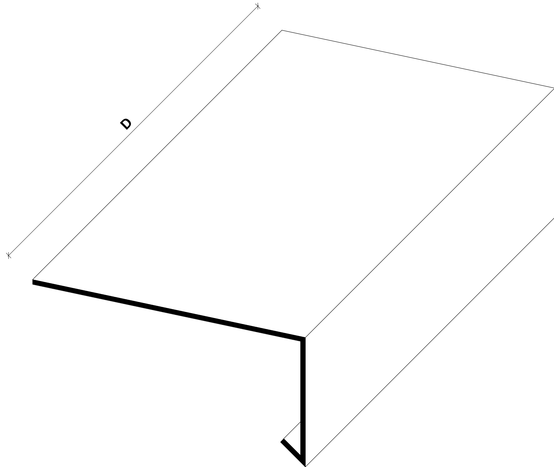
Sålbænk 1 3D 1:1
